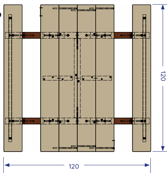
GP73-120 GP73GS-120
