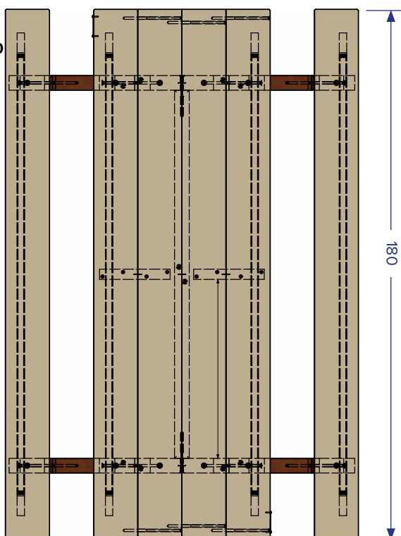
GP73-180 GP73GS-180
