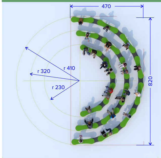
buitenarena 4 + 6 + 8 zitvlakken
