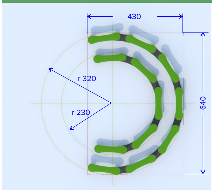
buitenarena 5 + 7 zitvlakken
