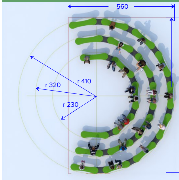
buitenarena 5 + 7 + 9 zitvlakken
