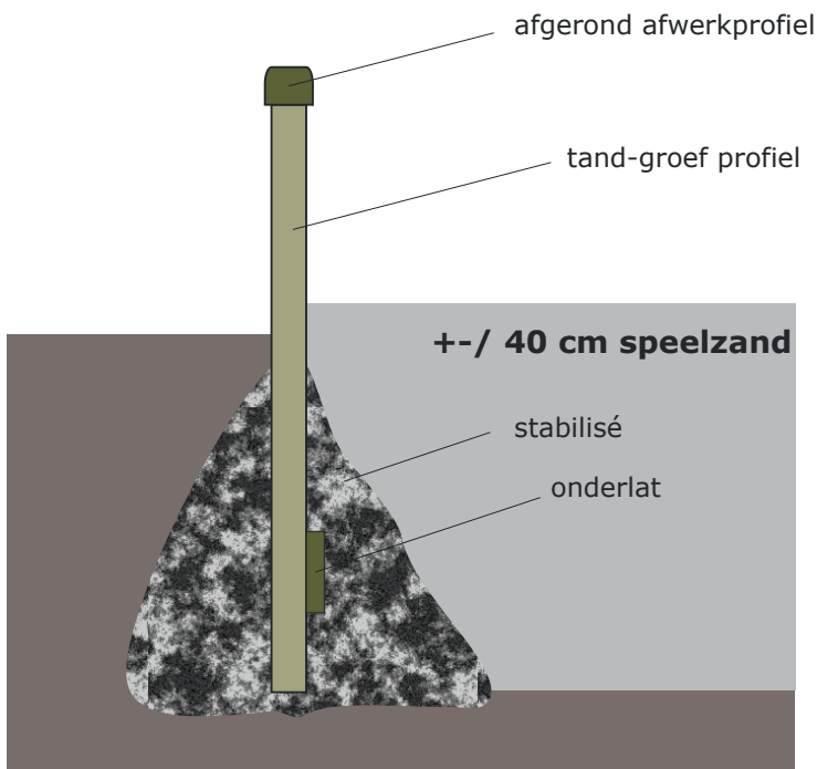
zand-cementmengeling („stabilisé“) schuin aanwerken
